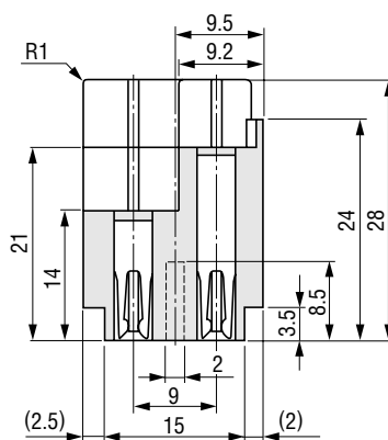
X-X' 断面図
